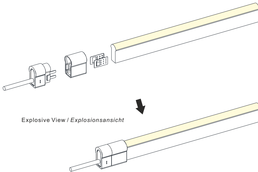
Finished Assembly View / Ansicht zusammengebaut.
